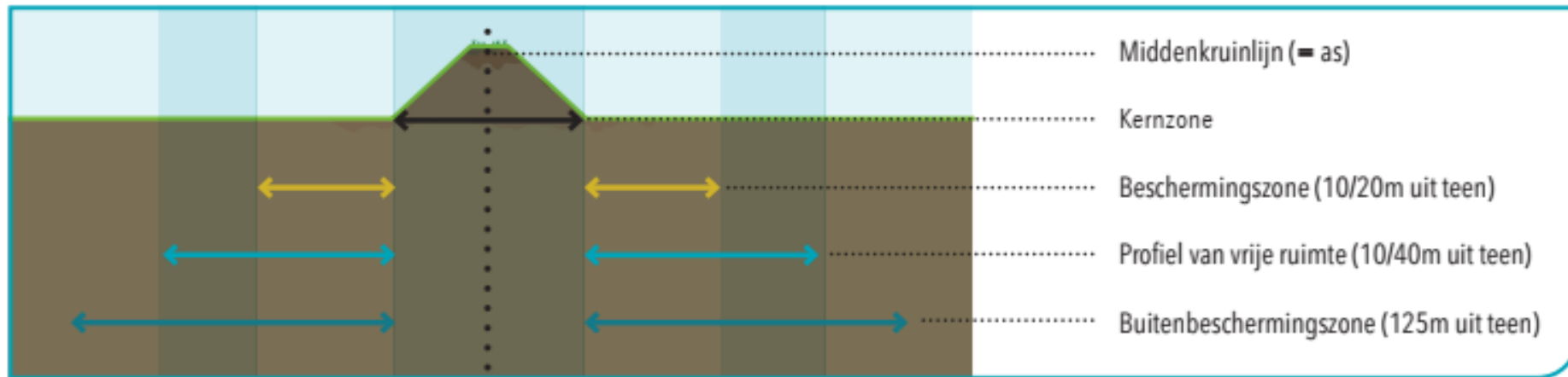
Schematische weergave zonerings waterkering
