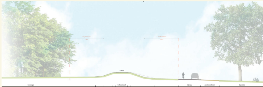
Dwarsprofiel 4 - 50jr
