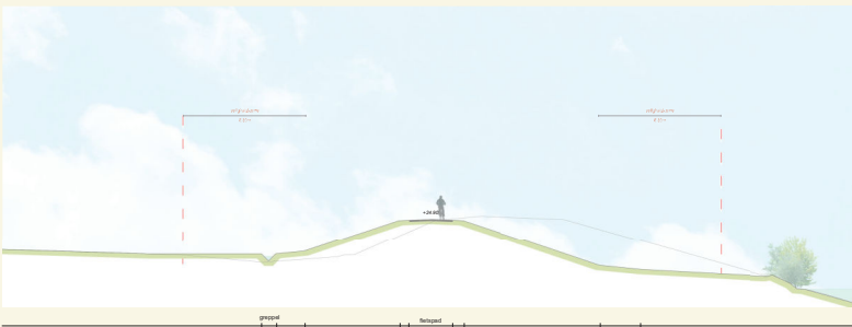
Dwarsprofiel 9 - 50jr
