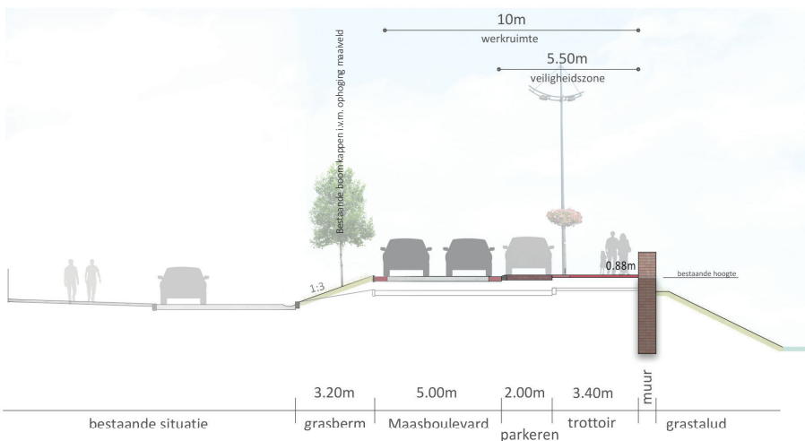
Doorsnede B: zichtjaar 2125 hoogte muur: 88 cm
