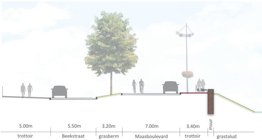
Doorsnede B: bestaande situatie hoogte muur: 36 cm
