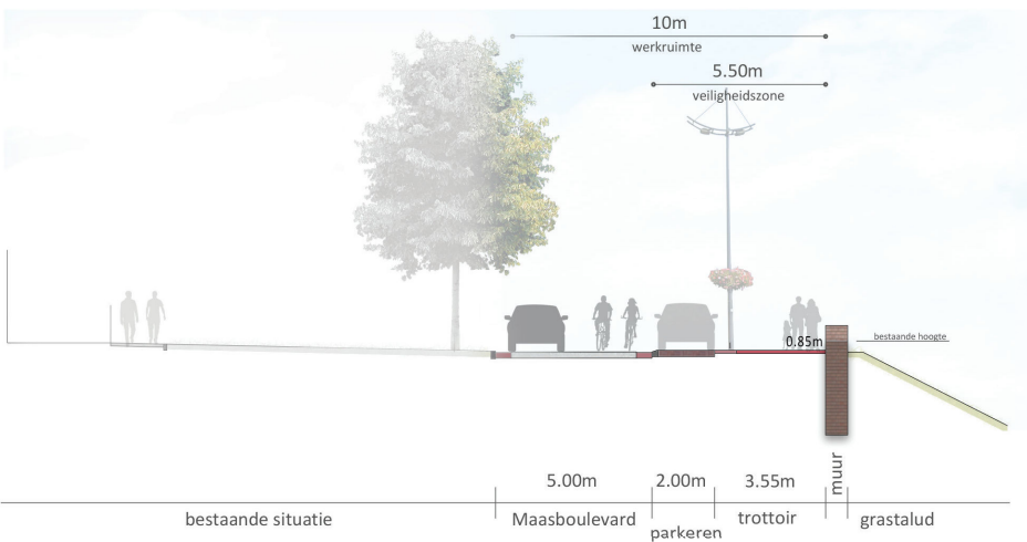
Doorsnede C: situatie tot 2075 hoogte muur: 85 cm
