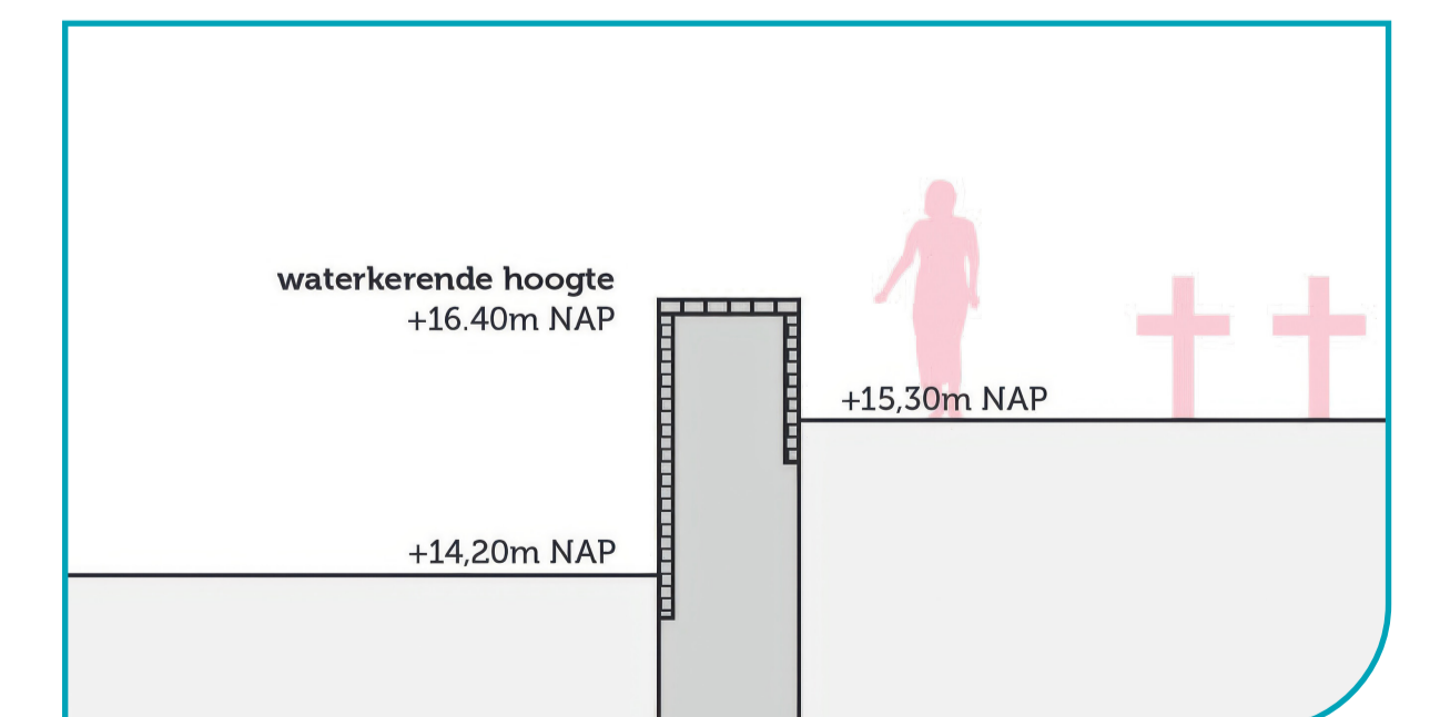
principeprofiel kering begraafplaats Nieuw Well
