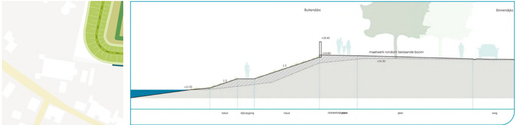
principeprofiel dorpsplein en demontabele kering
