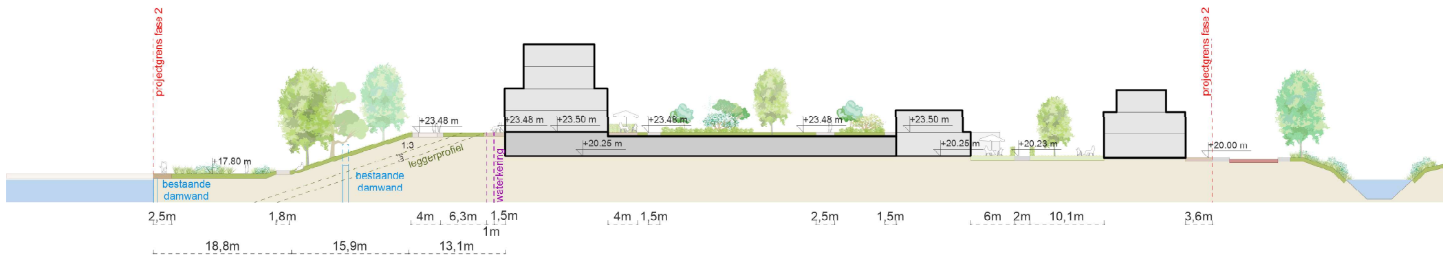
Principeprofiel B-B
