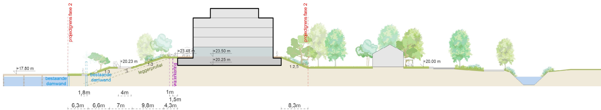
Principeprofiel A-A
